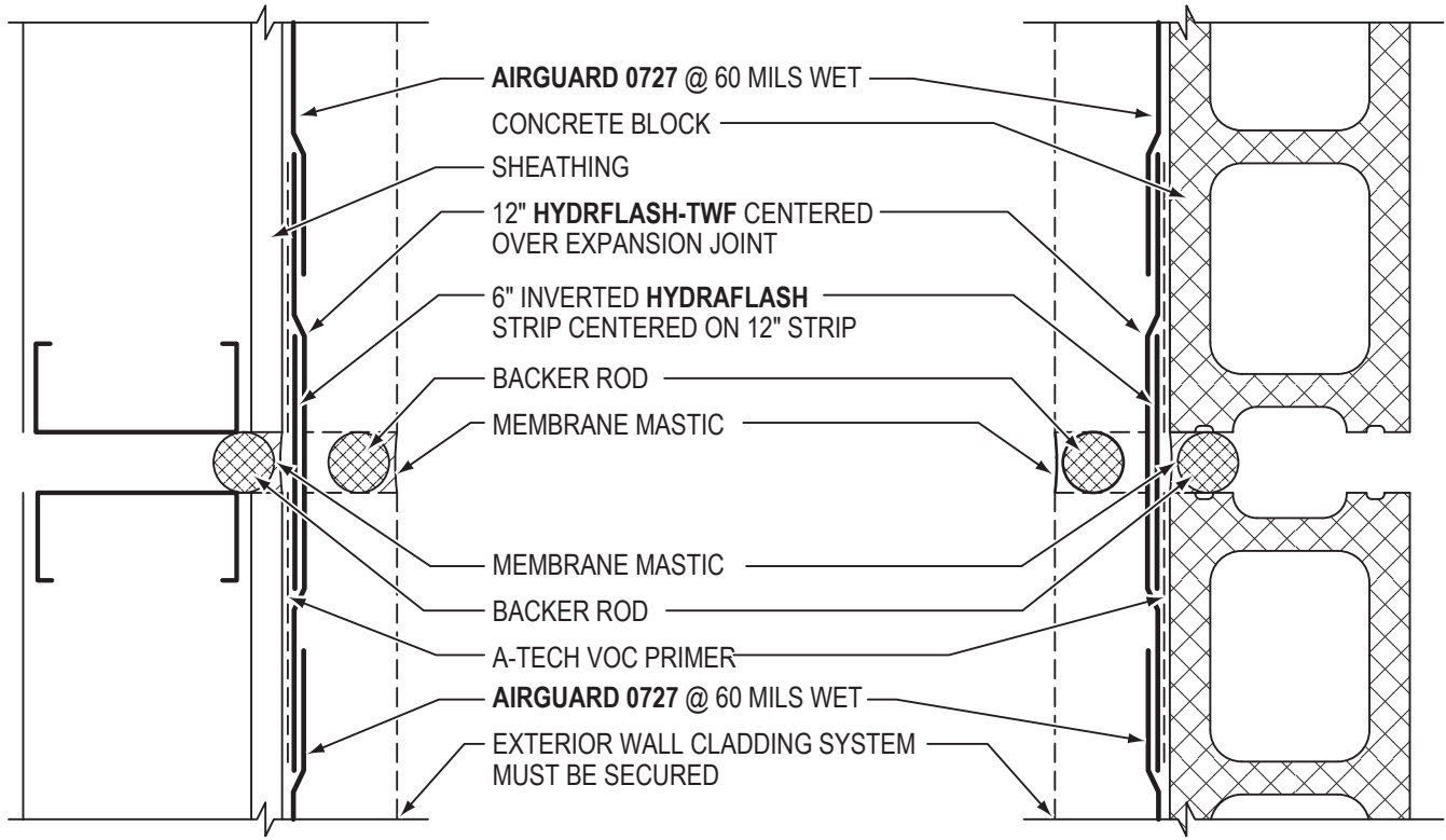
METAL STUD WALL
